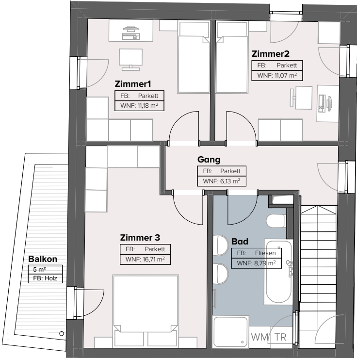
Obergeschoss
