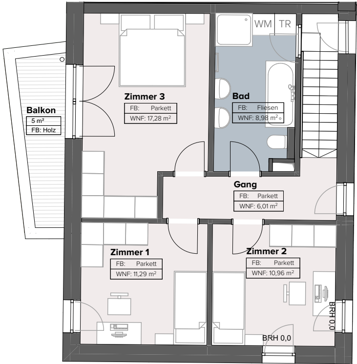
Obergeschoss
